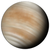
Venus
