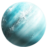
Uranus
